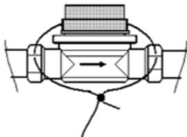
Рисунок 2 – Место пломбирования счетчика после монтажа на трубопровод.
