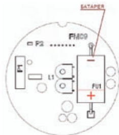
Рисунок А.2- Схема установки батареи питания на модуле электронном поз.4.
